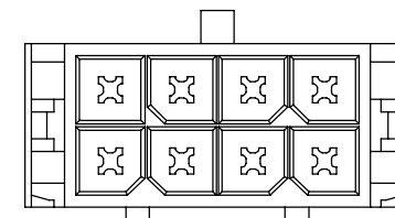
8-CKT
