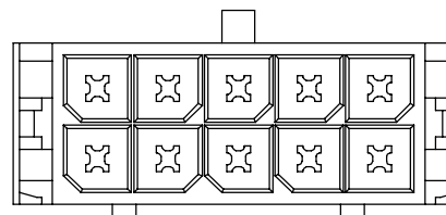
10-CKT
