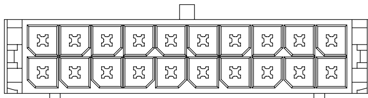
20-CKT
