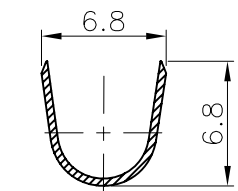
SECCION X-X
