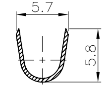
SECCION Y-Y
