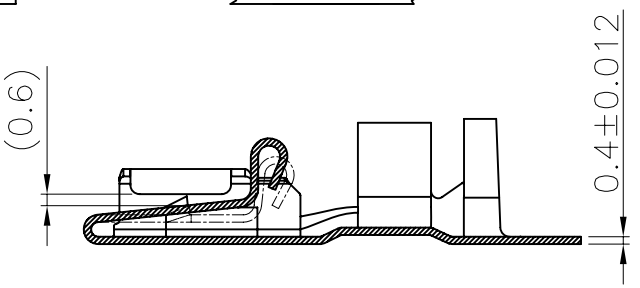
SECCION W-W
