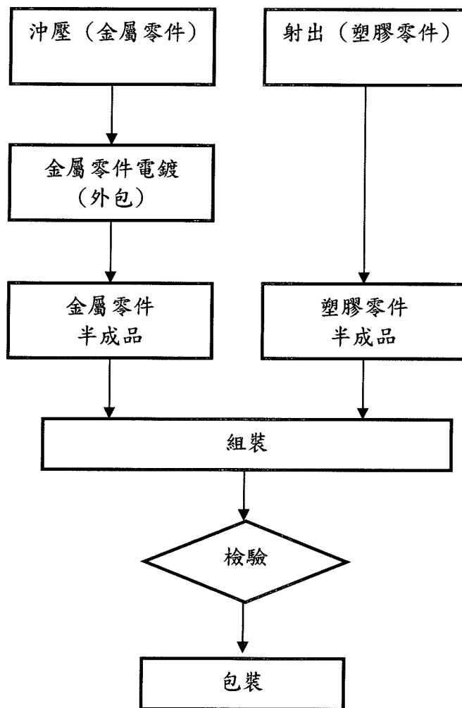
電子連接器製造流程圖
