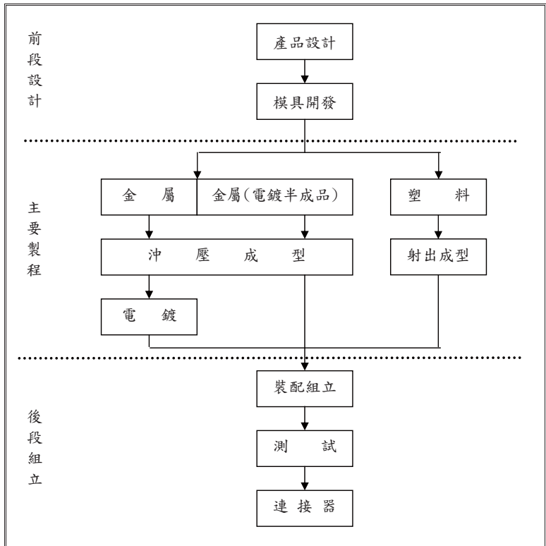
主要產品之製程圖
