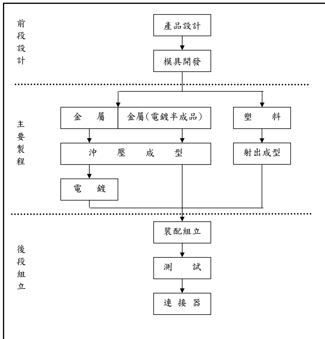
主要產品之製程圖
